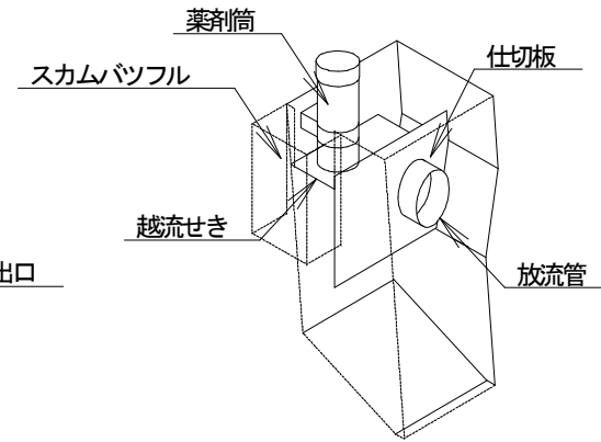
消毒槽立体図
