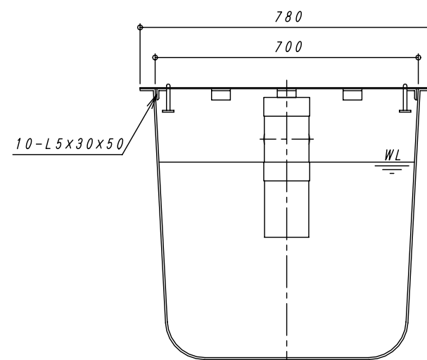
A矢視
