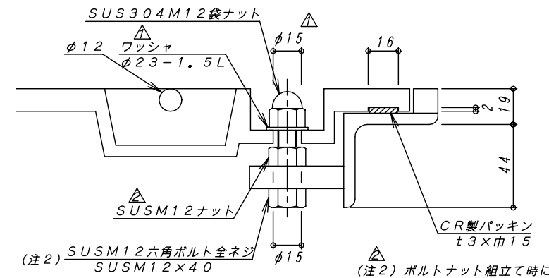
固定部詳細
