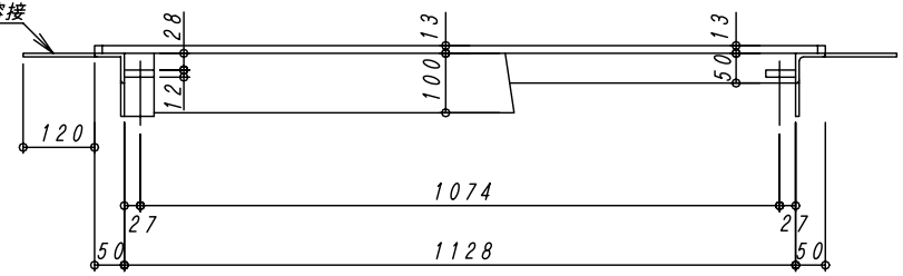
B-B断面図
