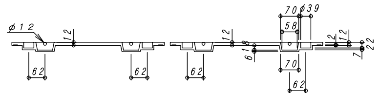
A-A断面図
