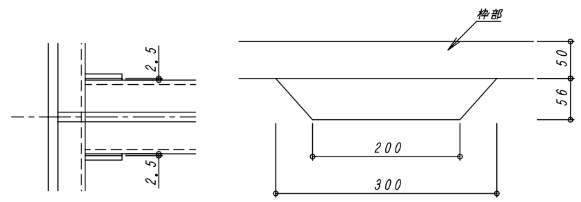
D部詳細
