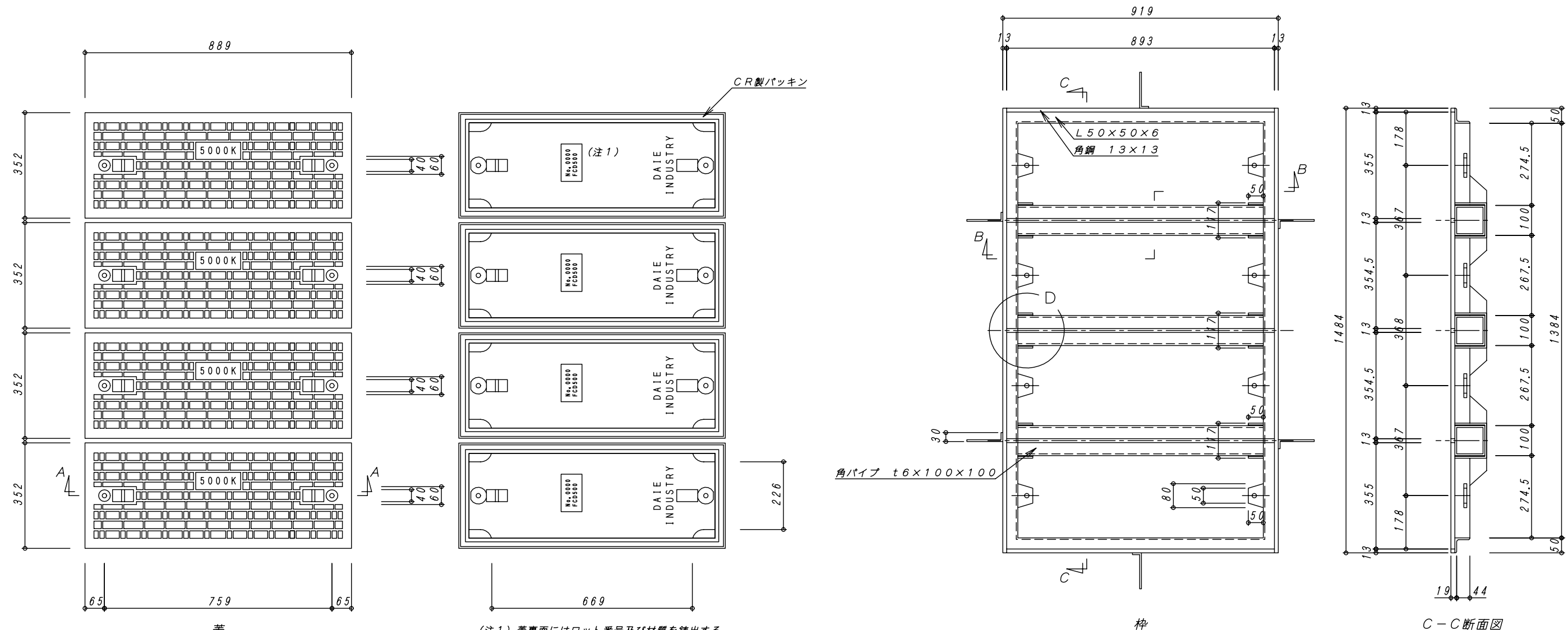
C-C断面図
