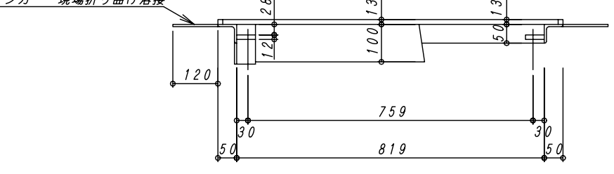
B-B断面図
