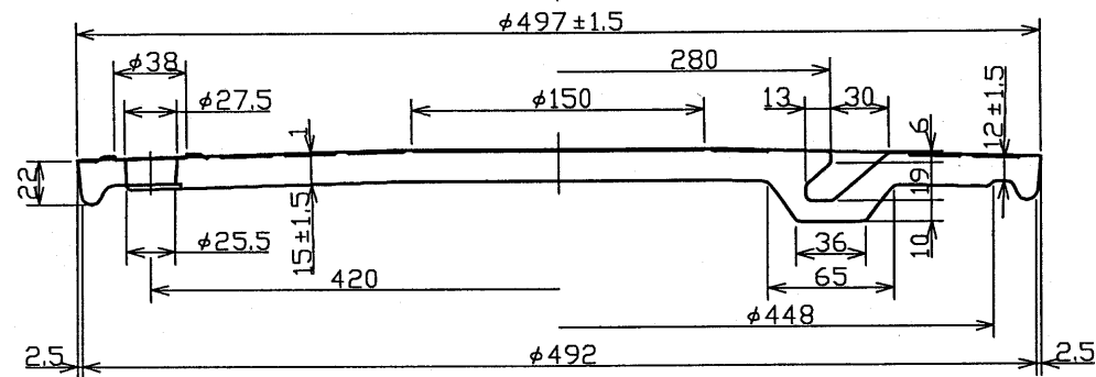
A-A断面
